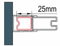
Profilé d'élargissement ACA1
